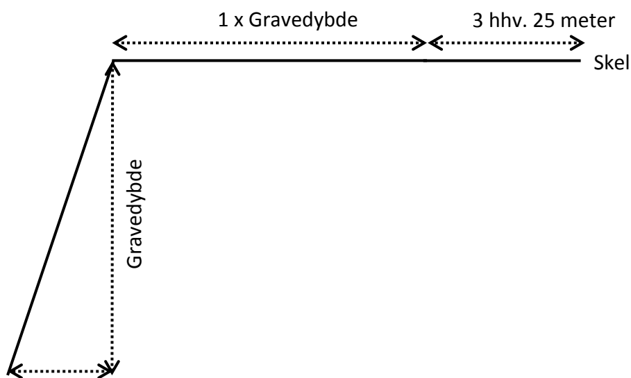
Figur 2. Principskitse for gravning nær skel/vej, hvis der graves stejlere end vilkår 15 og 17
