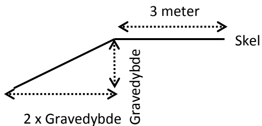
Figur 1. Principskitse for gravning nær offentligt vejskel
