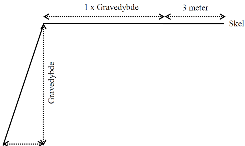
Figur 3 Principskitse for gravning nær skel/vej, hvis der graves stejlere end vilkår 17 og 19.
